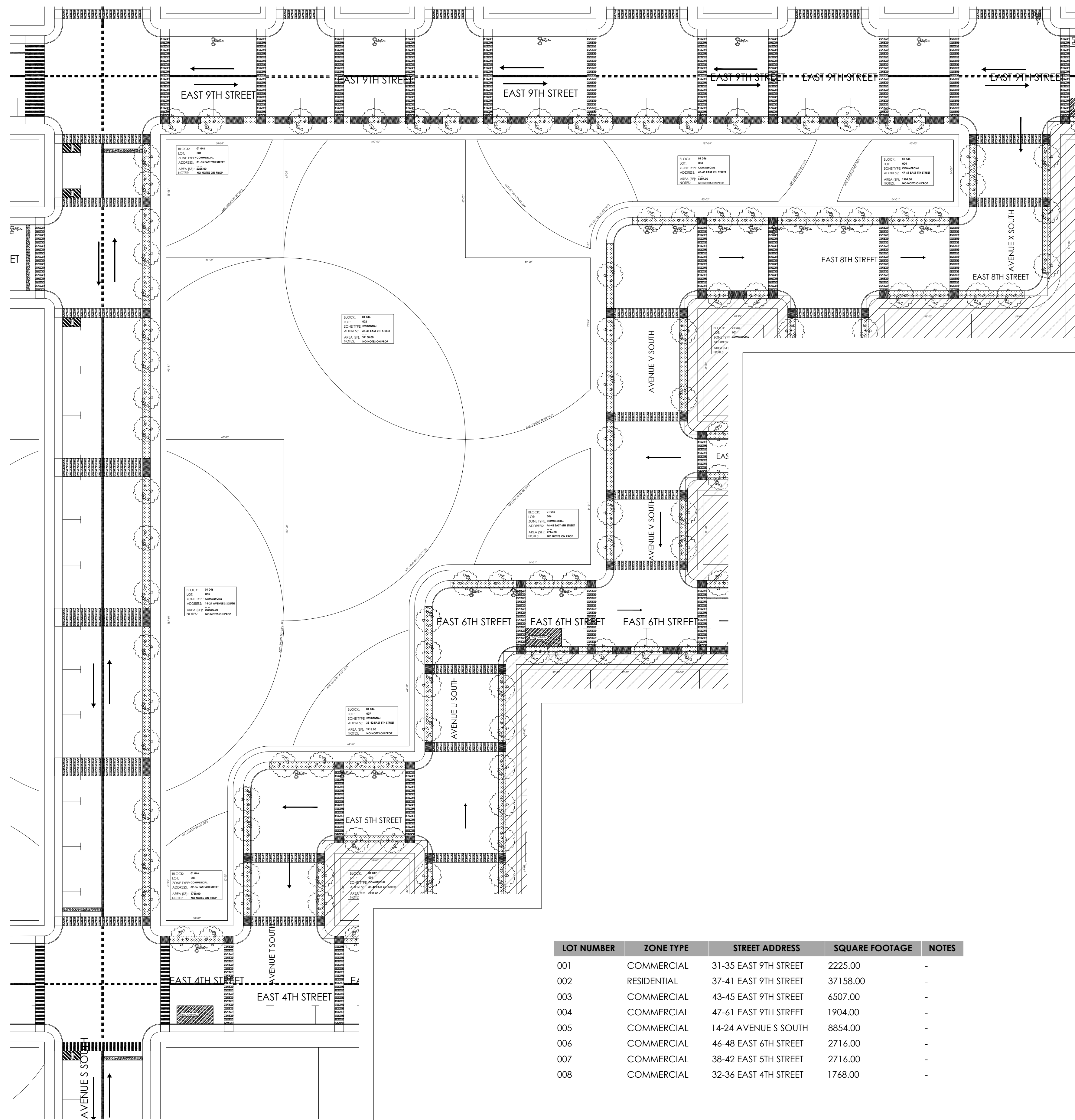
3 BLOCK 01 046 NORTHWEST VIEW G-004.101 SCALE: N.T.S
